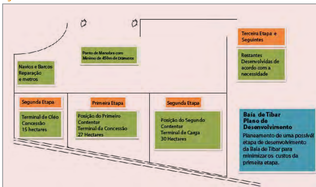
Figura 15 Plano de desenvolvimento do Porto de Tibar
